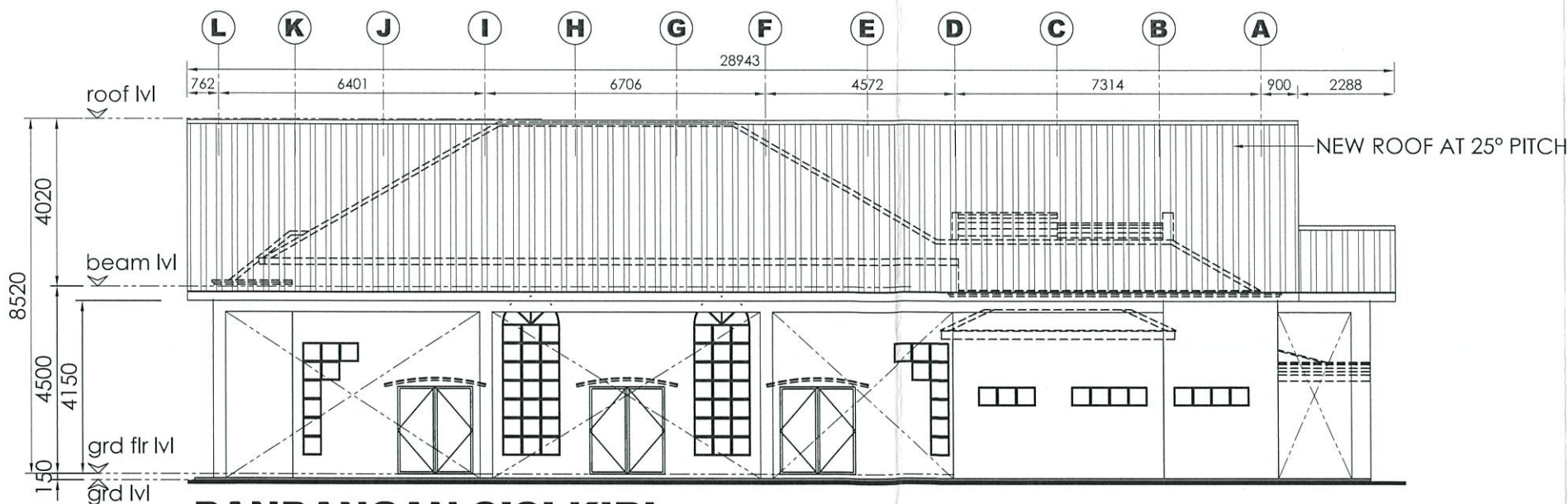
PANDANGAN SISI KIRI skala 1:150
