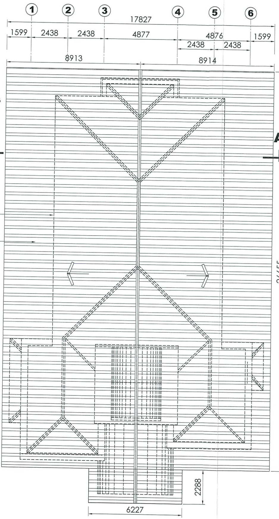
PELAN BUMBUNG skala 1:150
