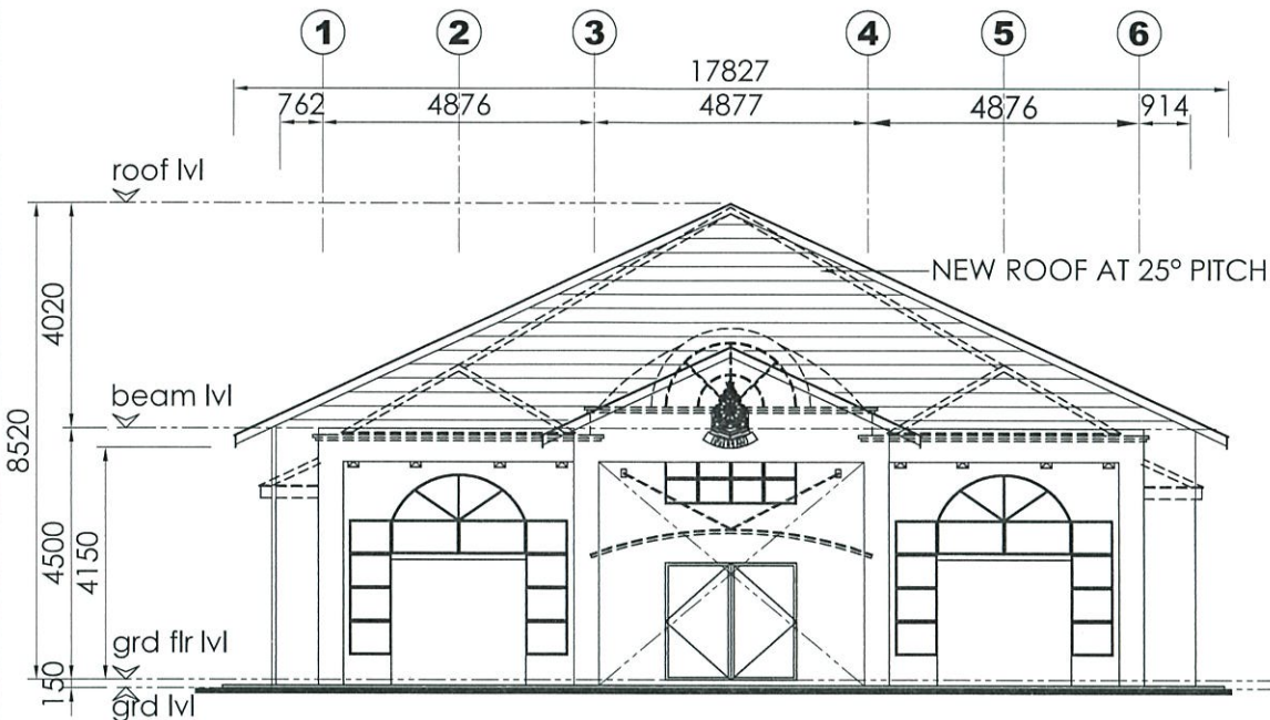
PANDANGAN HADAPAN skala 1:150
