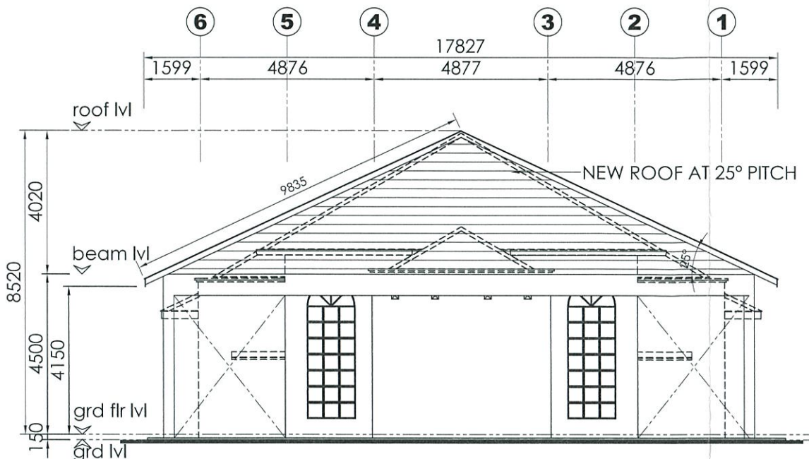
PANDANGAN BELAKANG skala 1:150
