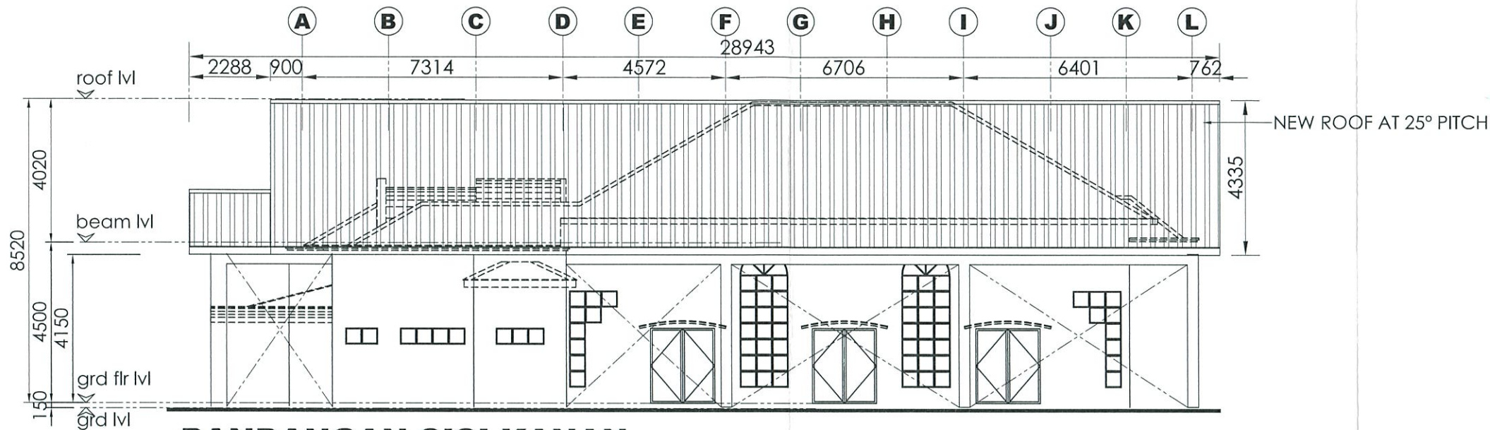
PANDANGAN SISI KANAN skala 1:150
