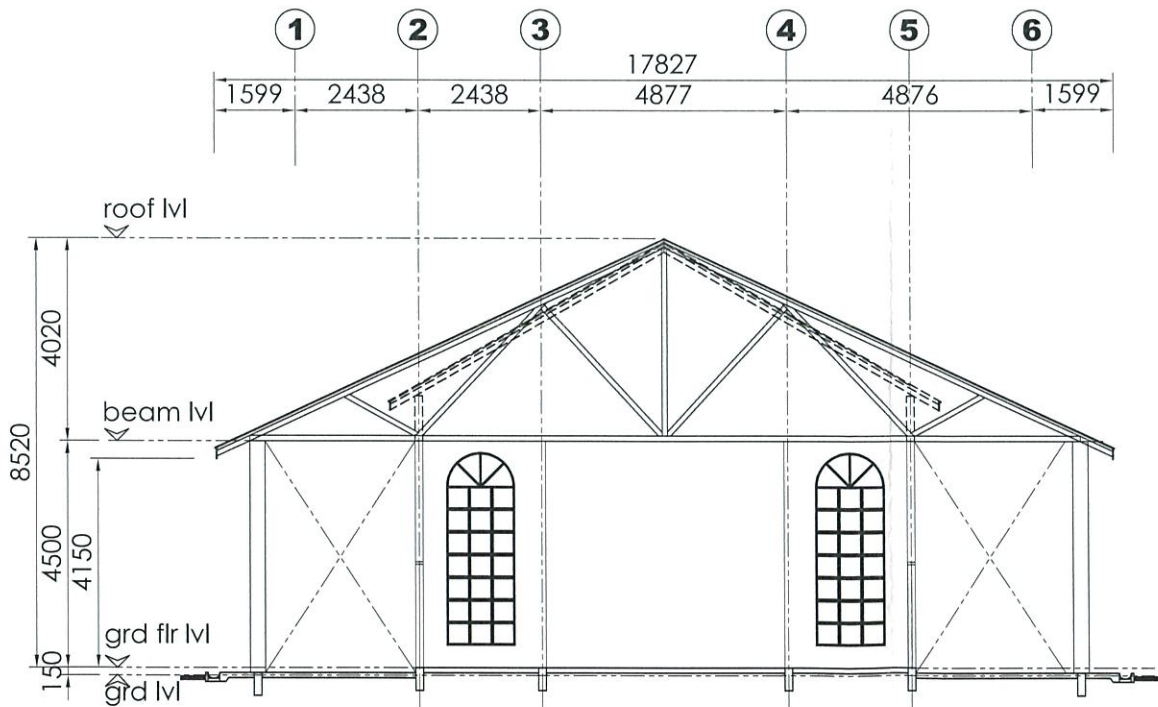
KERATAN A - A skala 1:150
