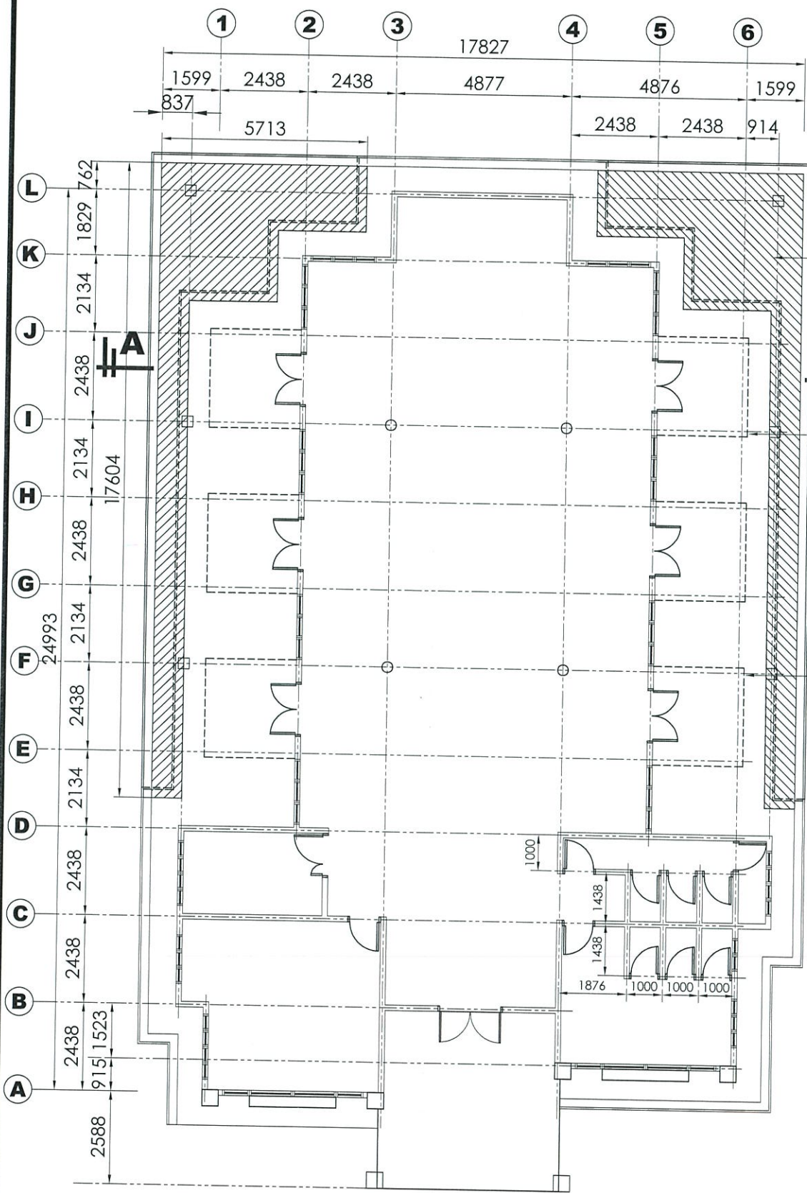
PELAN LANTAI skala 1:150
